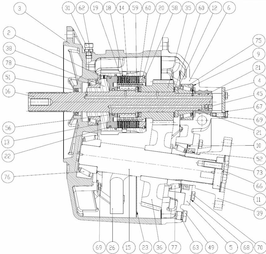
SEZIONE A-A
