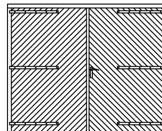
WGo2 2290 X 2000 (openslaand)
