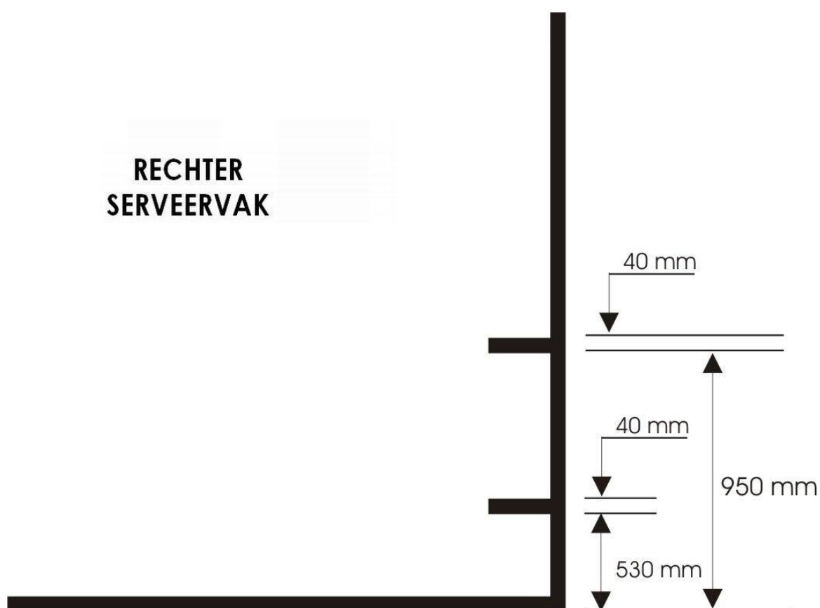
FIGUUR G: EVENTUELE MERKTEKENS VOOR SHUTTLETEST OP ENKELBAAN
