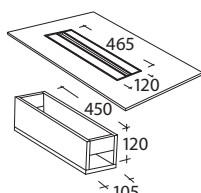
TKB1 Kabelgenomföring med elbrunn Cable slot with box
