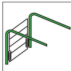
Trekveren veer-in-veer
