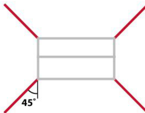
fig. 2 Bovenaanzicht vrijstaand
