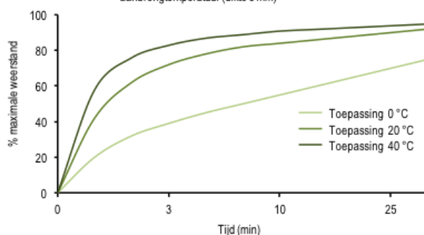
Reactiesnelheid versus aanbrengtemperatuur (dikte 5 mm)
