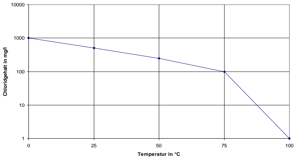
Abbildung 7: zulässiger Chloridionengehalt in Abhängigkeit von der Temperatur
