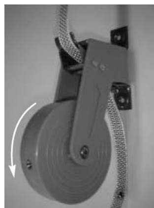
Draai de veer voldoende op spanning. Houdt deze spoel goed vast i.v.m.de grote veerspanning.
