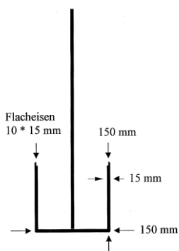
Ankermixer, art.nr. 4249
