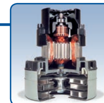
TwinFlo zuigmotor
