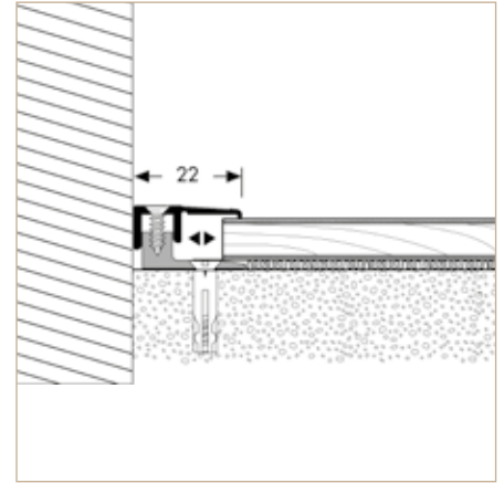
Schraub Endprofilprofil 6,5–16 mm (bis 26 mm mit Lift up Block)
