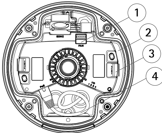
1 ファンコネクタ
