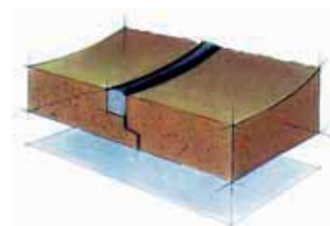
Principe van de veiligheidsvoeg (SF)
