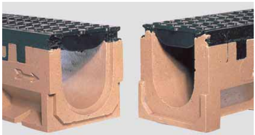
Veiligheidsvoeg (SF) opvullen met elastisch blijvende voegmassa.
