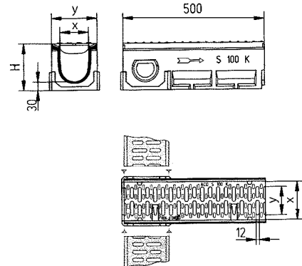
Gootelement, 0,5 meter, voor hoek-, T- en kruis verbindingen
