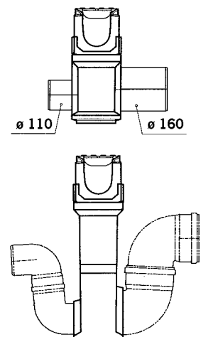
Aansluiting met stankslot (S100K)
