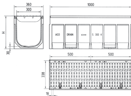
Gootelement S300K.
