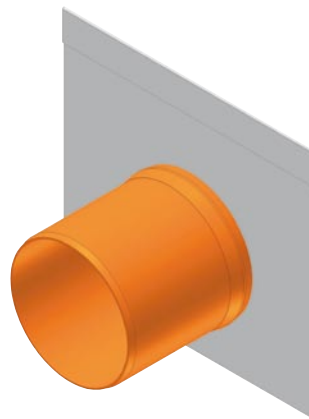
eindplaat met horizontale PVC-uitloop DN 200, verzinkt staal, type 010
