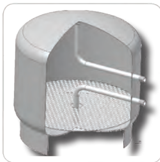
Lochblech/Trennblech in jeder Speichergröße möglich
