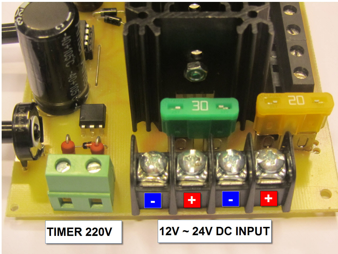
Fig2: Aansluiting klok en Voedings spanning
