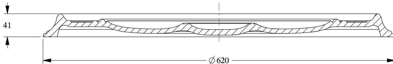
SECTION A-A
