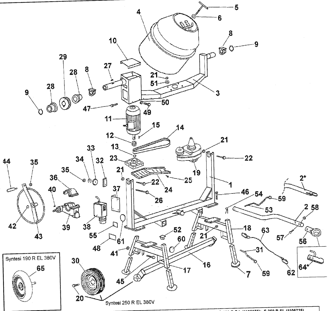
TAV. 1 - BETONIERA - BETONNIERE - CONCRETE MIXER - BETONMISCHER - HORMIGONERA : S 190 R E L (1105675); S 250 R EL (1105725)
