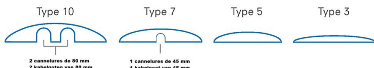
Modèles disponibles des ralentisseurs Slowly
