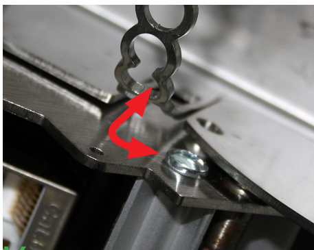
✓ Richtig / Right Schraube kann unter der Lasche wegtauchen. / Please ensure the metal strap is bent back, allowing the screw to move properly.
