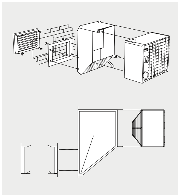
Fig. 2: doorsnede en zijaanzicht van de Cat met mengkamer.
