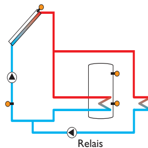
Uitvoering pomp
