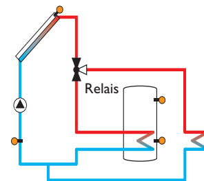
Uitvoering klep
