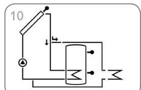
Standaardzonnestelsysteem met restwarmteafvoer (pagina 43)
