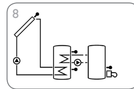
Zonnestelsysteem met naverwarming door vaste-brandstofketel (pagina 34)
