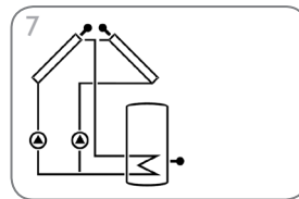
Zonnestelsysteem met 2 collectoren en 1 boiler (pagina 31)
