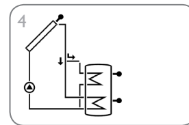
Zonnestelsysteem met gelaagde buffering (pagina 22)
