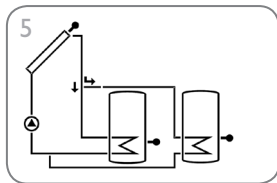
Zonnestelsysteem met 2 boilers met kleplogica (pagina 25)
