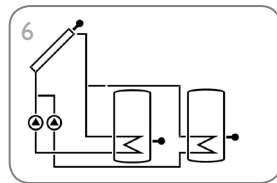
Zonnestelsysteem met 2 boilers met pomplogica (pagina 28)
