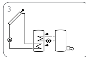
Zonnestelsysteem met naverwarming (pagina 17)
