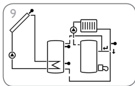
Zonnestelsysteem met verwarmingscircuit-retourverhoging (pagina 40)
