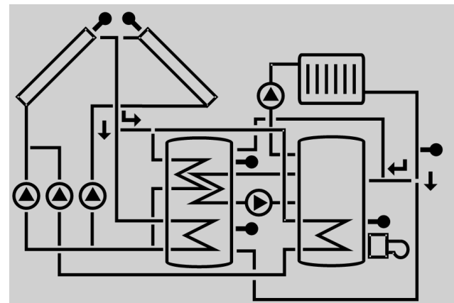
Collectoren met collectorsensor
